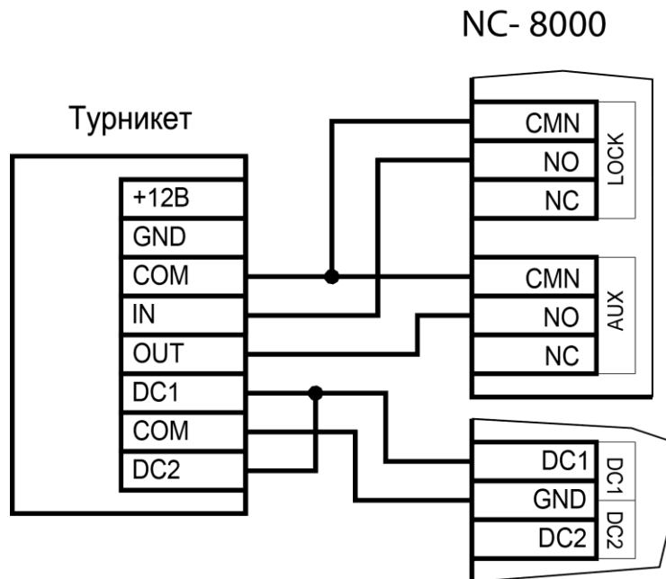
Рисунок 14. Схема подключения контроллера к турникету
