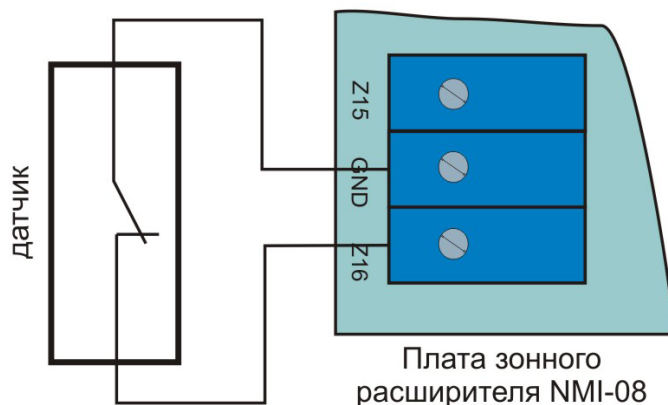
Рисунок 2(б). Подключение охранного датчика с двумя состояниями.
